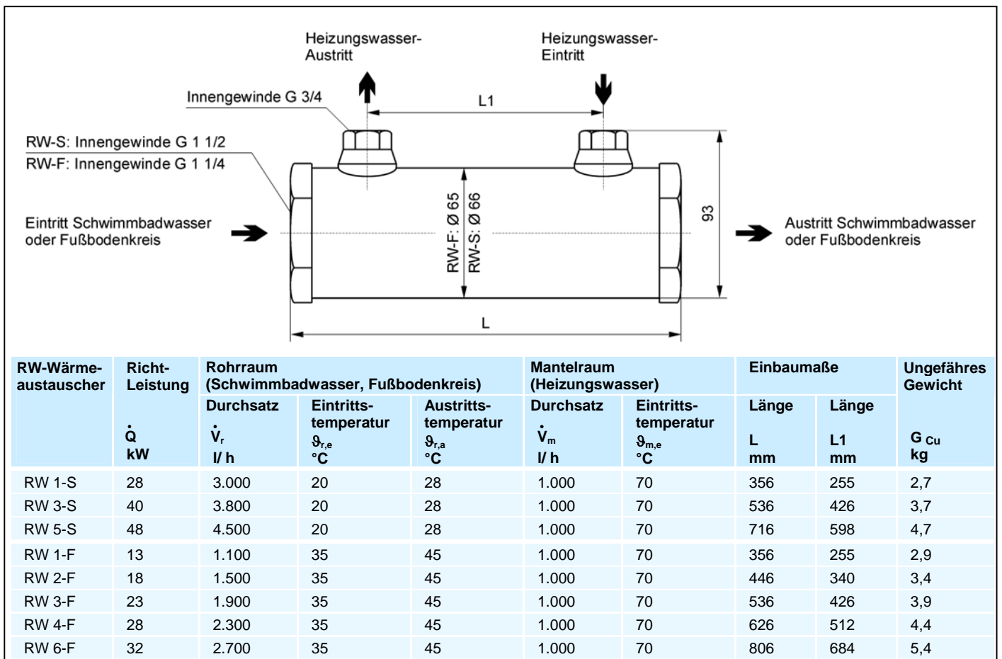
Bild 2: Abmessungen und Richtleistungen der Rohrbündel-Wärmetauscher Ausführungen RW-S und RW-F
