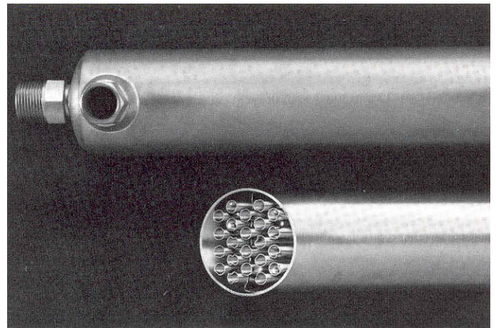
RW-Wärmetauscher aus Kupfer oder Kupfer-Nickel
