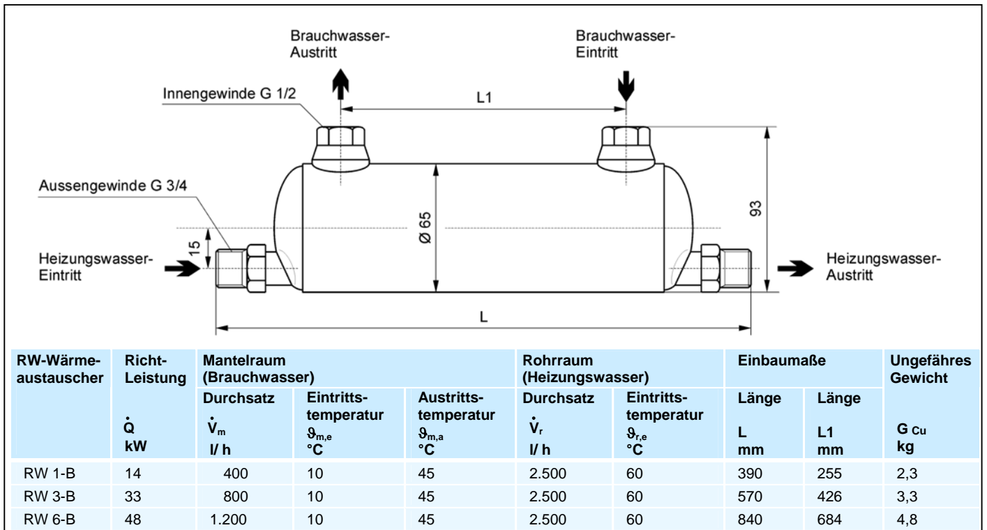
Bild 1: Abmessungen und Richtleistungen der Rohrbündel-Wärmetauscher Ausführung RW-B
